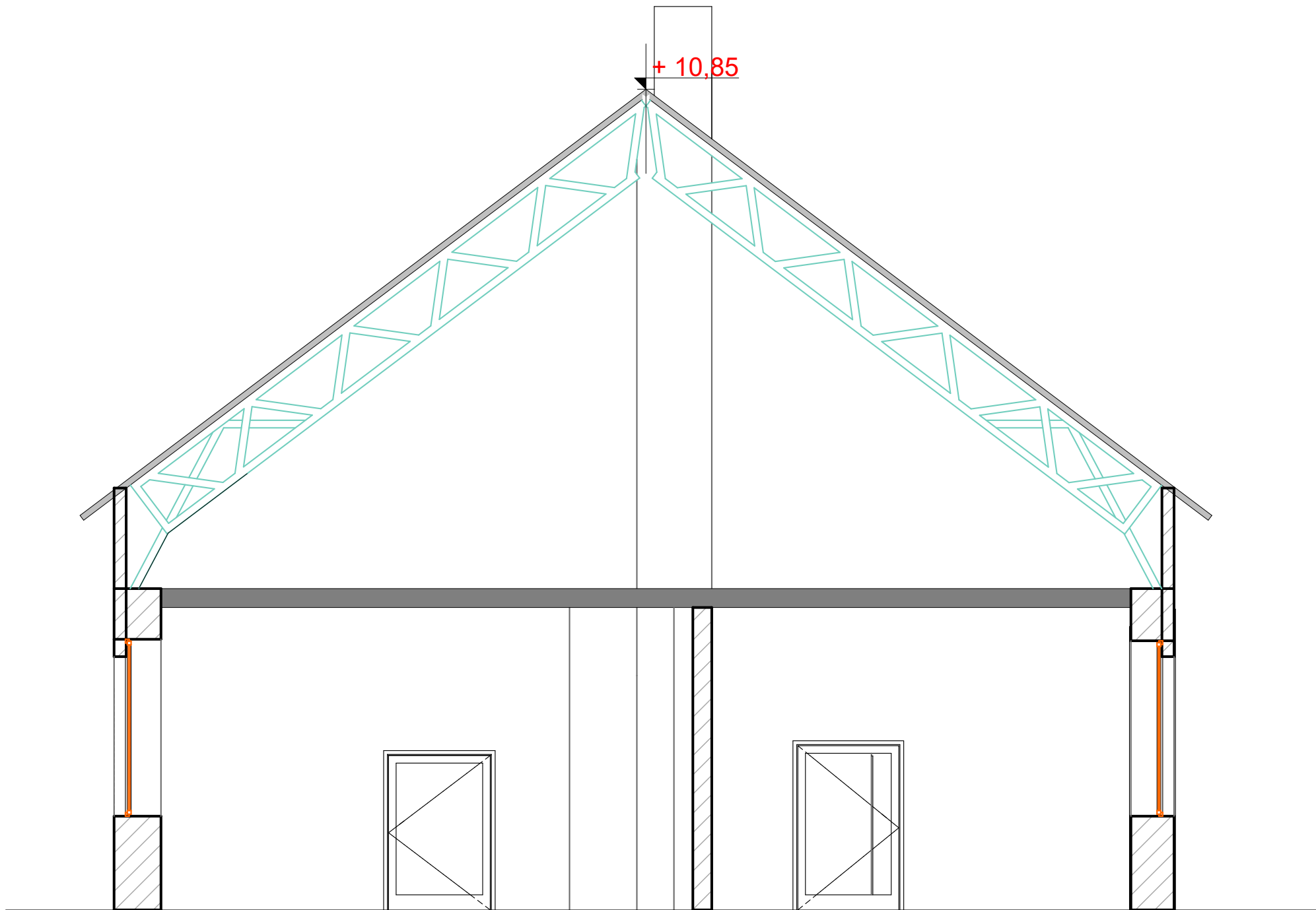
PRZEKRÓJ
